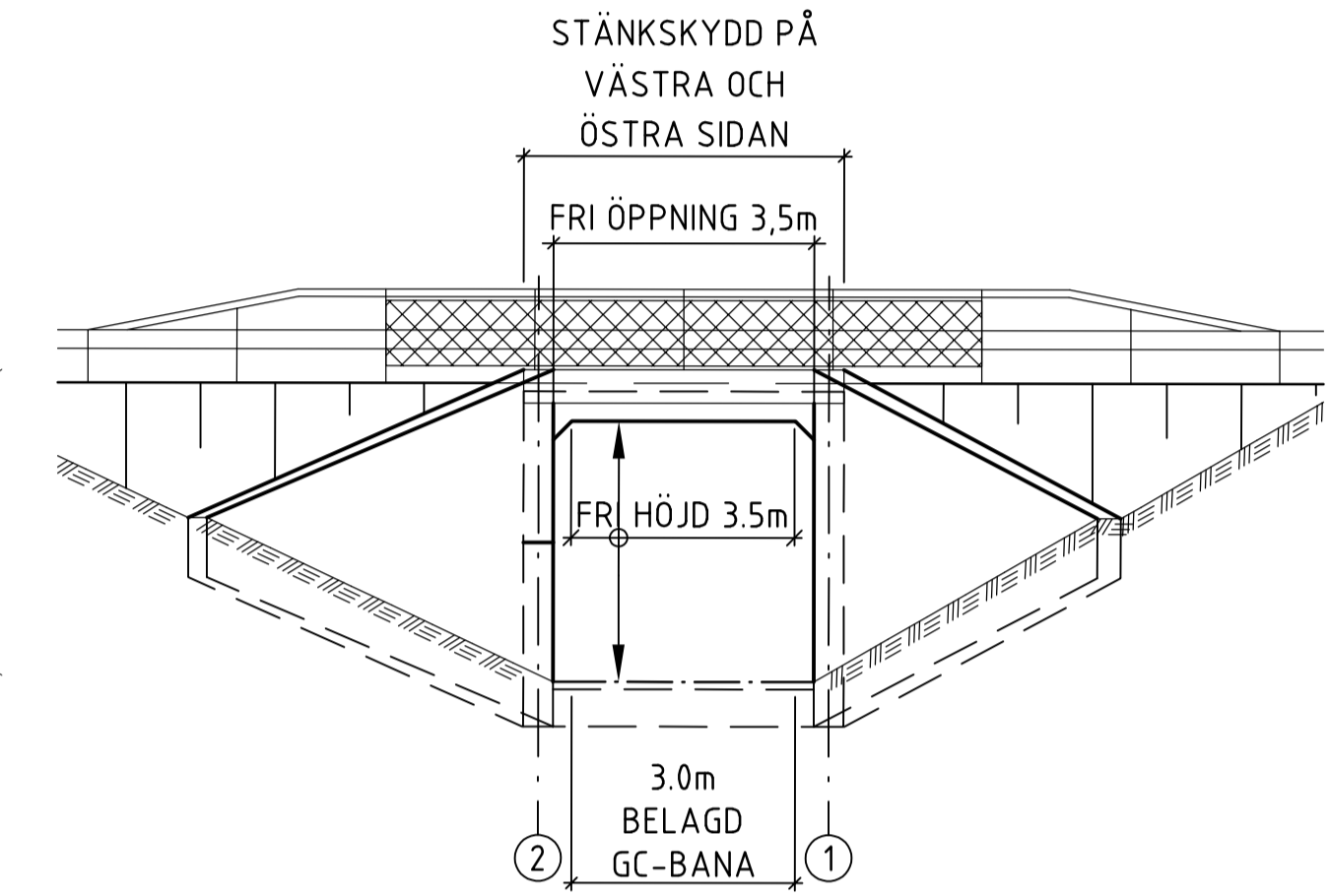
SEKTION B-B 1:100
