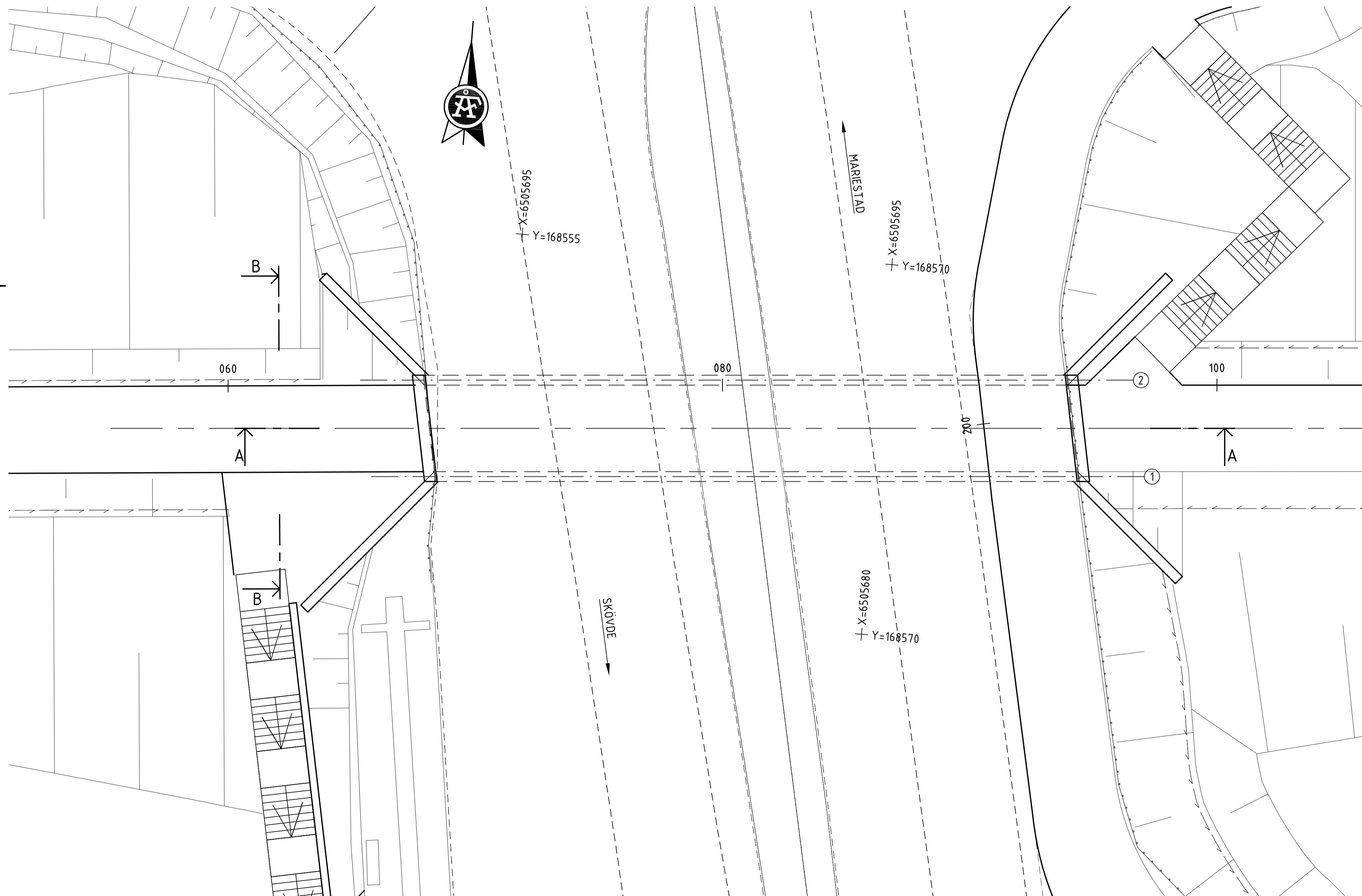
PLAN 1:100
