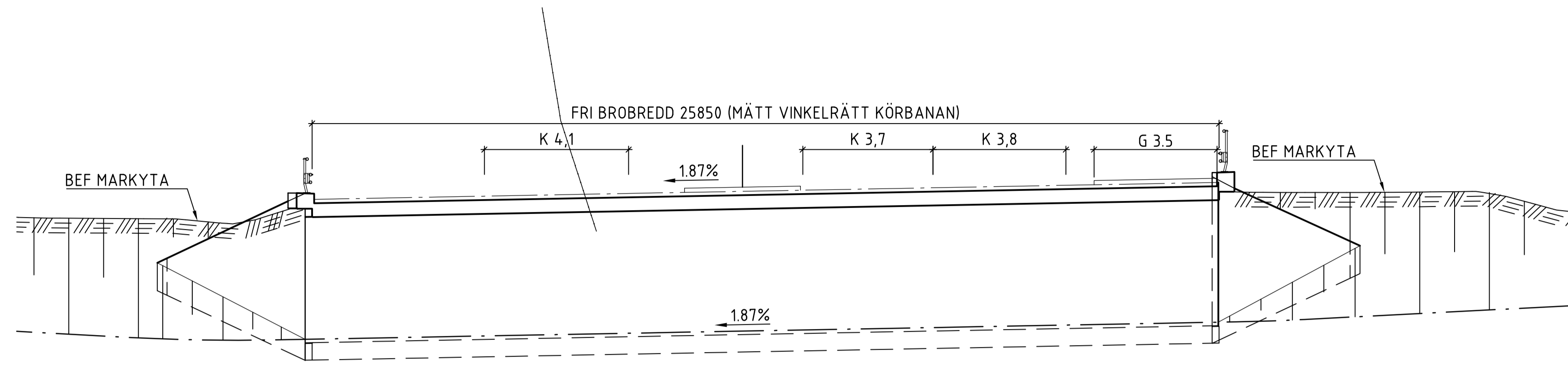
SEKTION A-A 1:100
