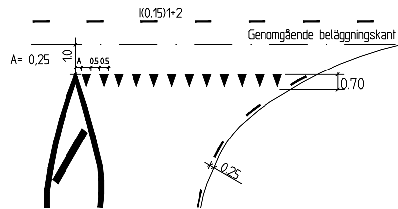
DETALJ 1
