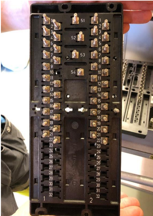
Modell ny JAZ-plint med tunna fjäderstift som är utpressade för låsning. Här gäller att se upp, så att inte stiften har åkt ut efter reläbyte. Denna nya typ av plint är den som är behäftad med ovanstående beskrivna problem.
