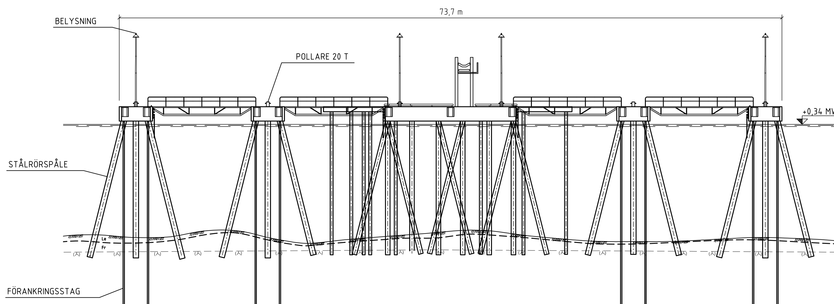
ELEVATION A-A 1:200
