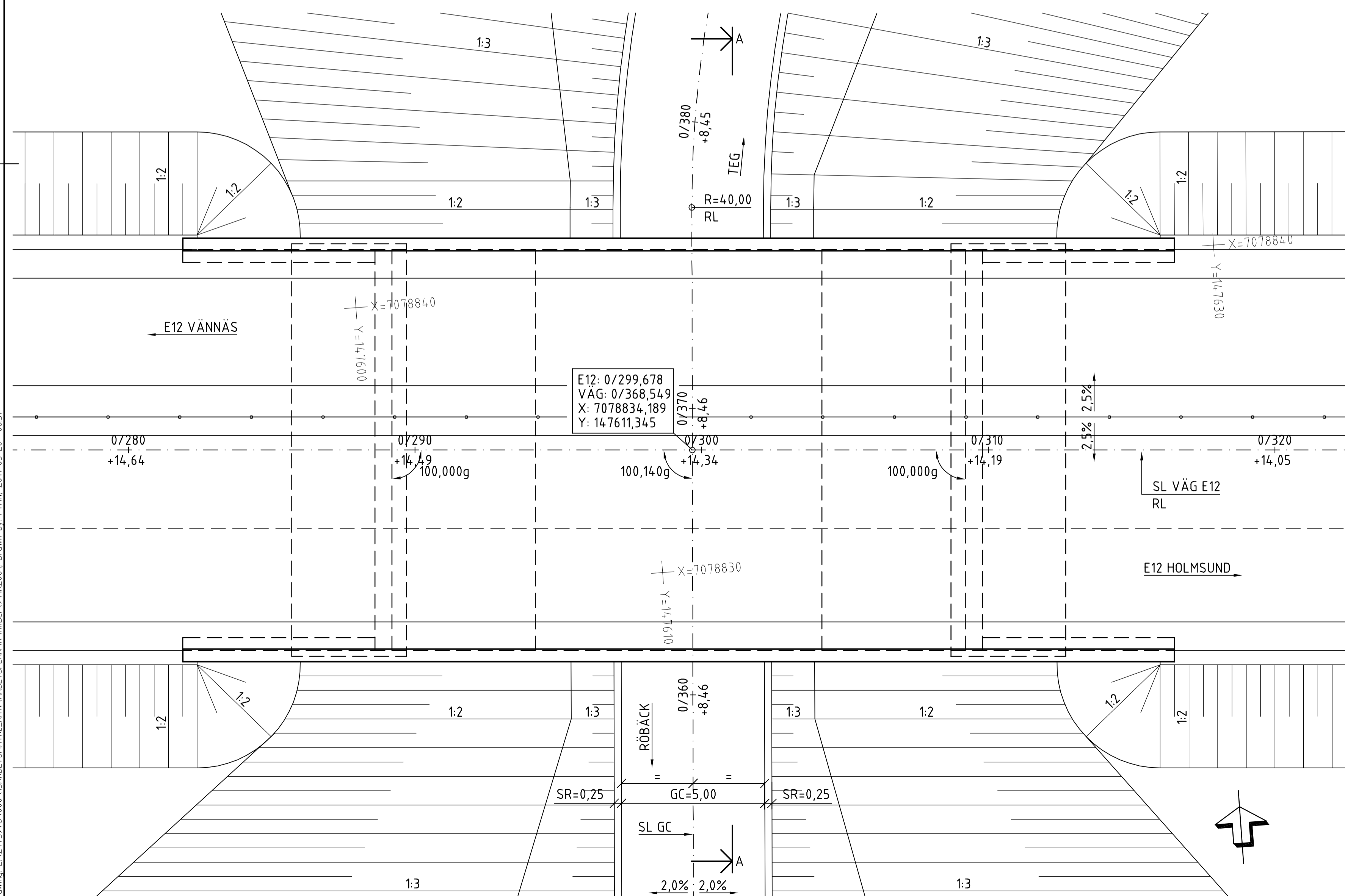
PLAN SKALA 1:100
