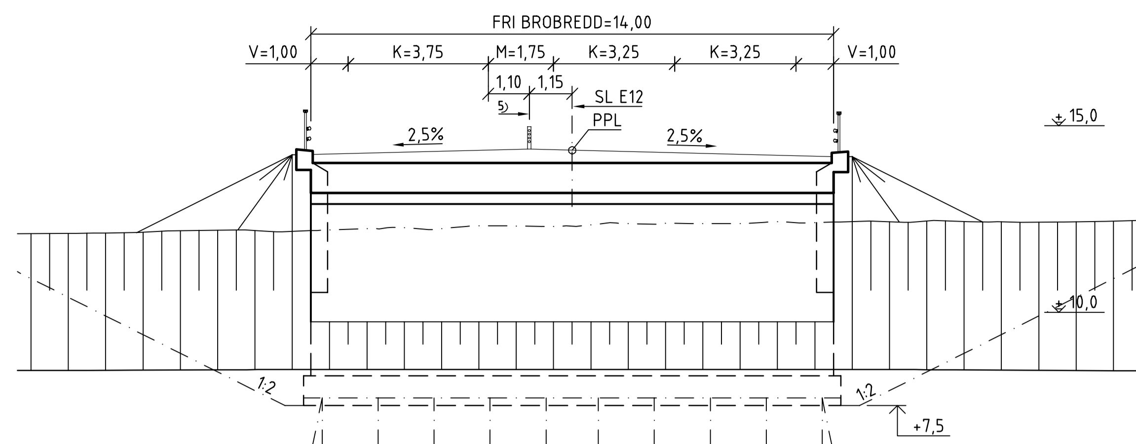
SEKTION A SKALA 1:100 3) CL RÄCKE/BOMBERING ÖK BELÄGGNING
