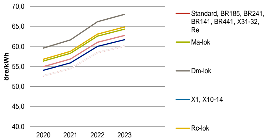
Prisindikator drivmotorström 2020-2023
