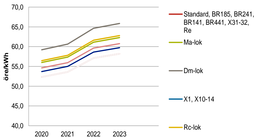
Prisindikator drivmotorström 2020-2023
