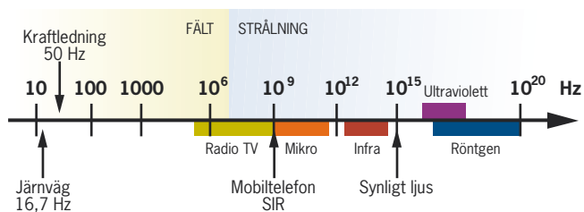
Elektromagnetiska spektrumet
